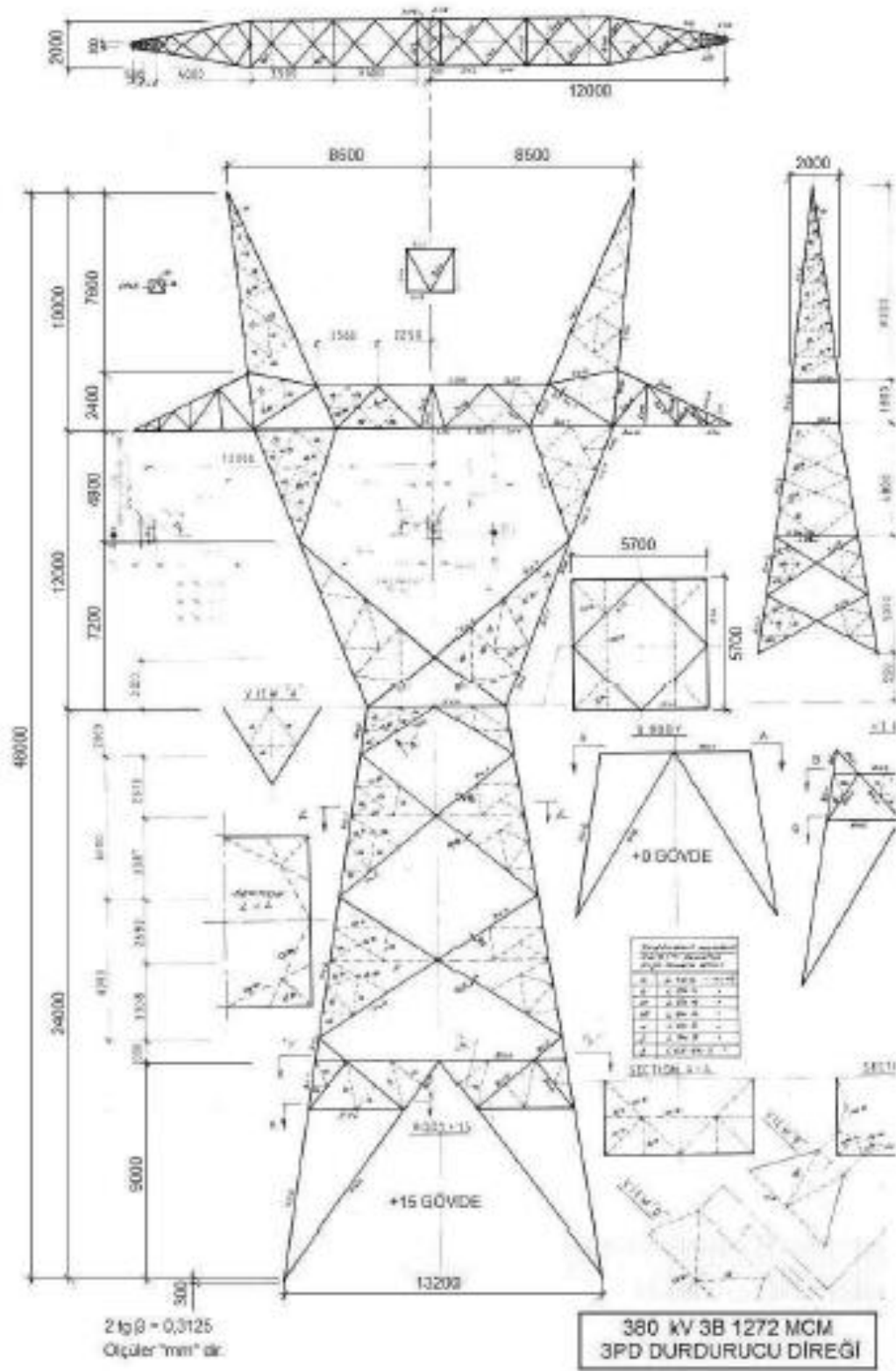
Şekil A.8. 380 kV 3B (üçlü demet) 3PD tek devre direği
