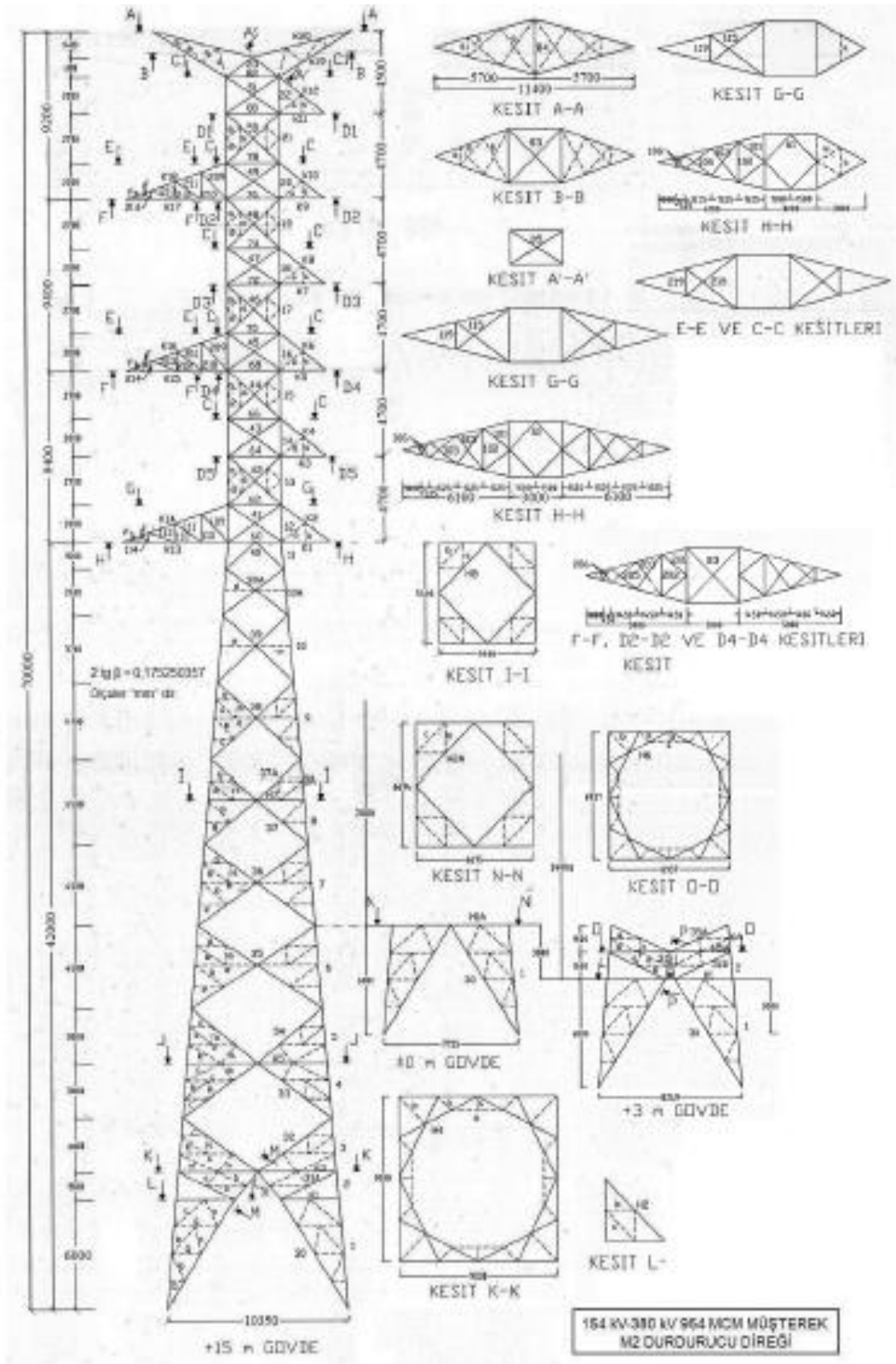
Şekil C.5. 380 kV 954 MCM 380/154 müşterek M2 direğinin ana ölçülerinin gösterimi
