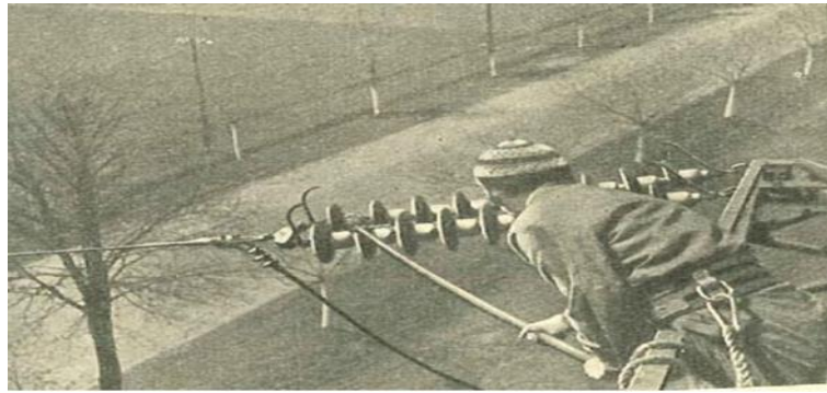
Şekil 2.2. 1935 yılında Polanya’da yapılan bir canlı çalışma [11]
