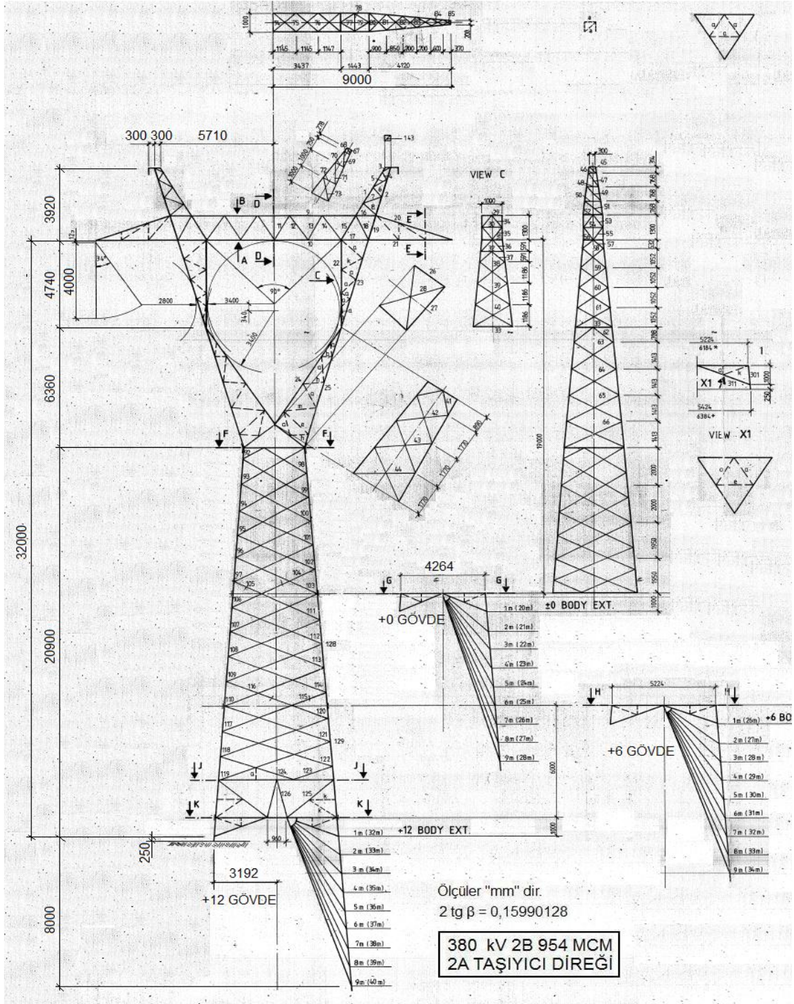
Şekil A.2. 380 kV 2B (ikili demet) 2A tek devre direği
